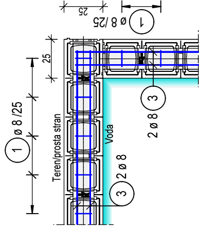
TLORIS M1:25 DETAIL KOTA
